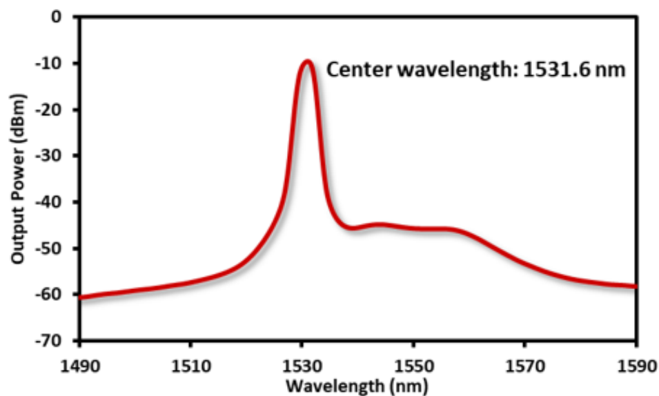
Fig. 2. Output spectrum
